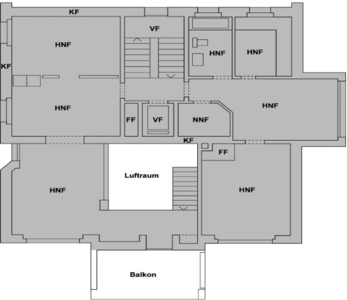
Grundriss 1. Obergeschoss:
