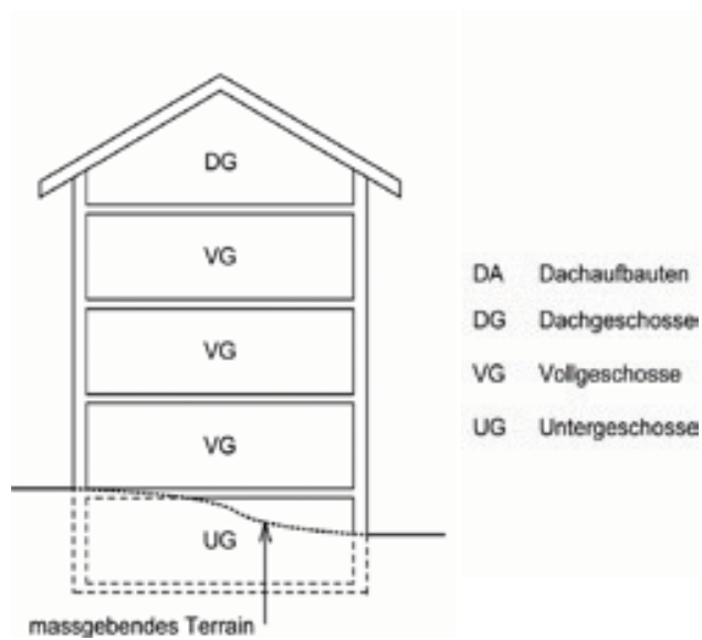
Skizzen zur Definition Vollgeschoss gemäss BMBV vom 25. Mai 2011
