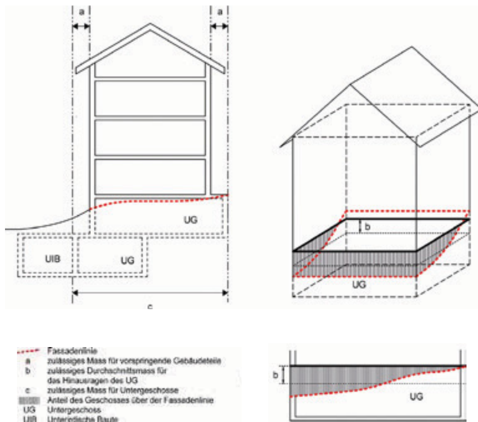
Skizzen zur Definition Untergeschoss gemäss BMBV vom 25. Mai 2011
