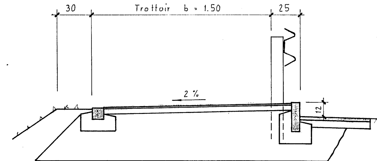
Trottoir mit Leitplanke
