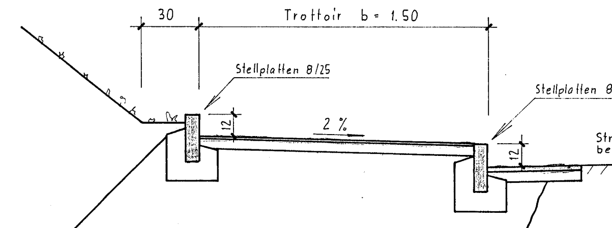
Trottoir mit Stellplatte
