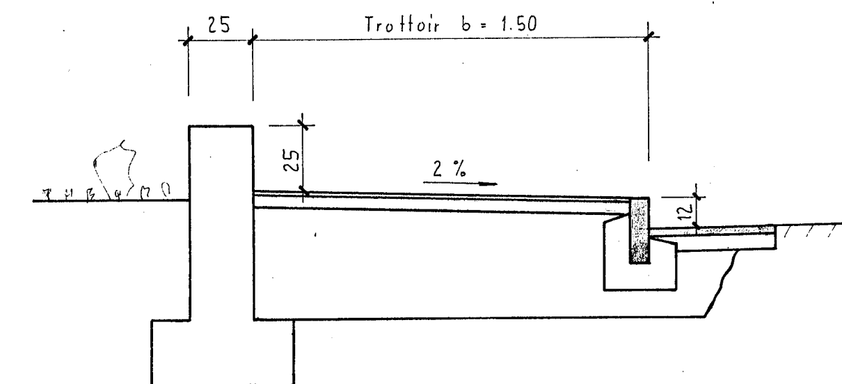
Trottoir mit Sockel
