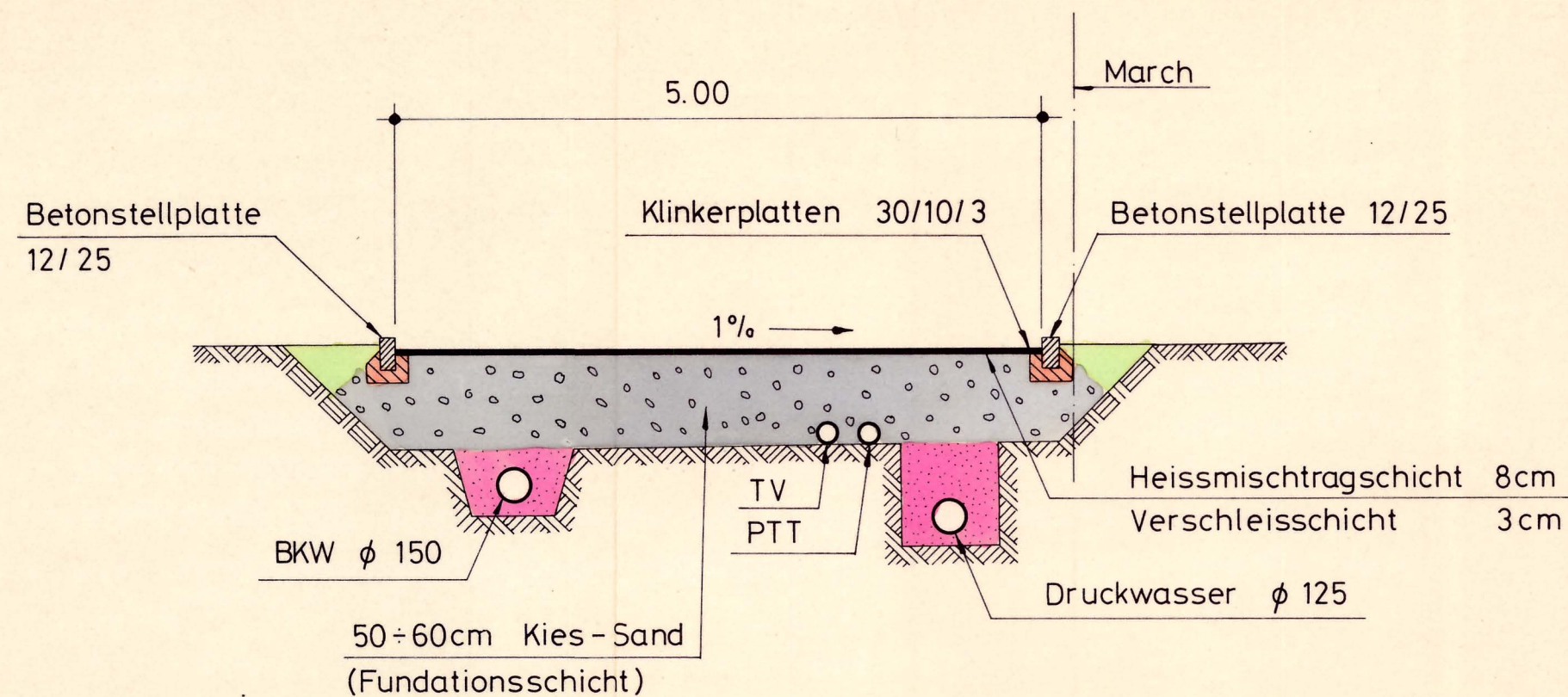
Querprofil 2 1:50
