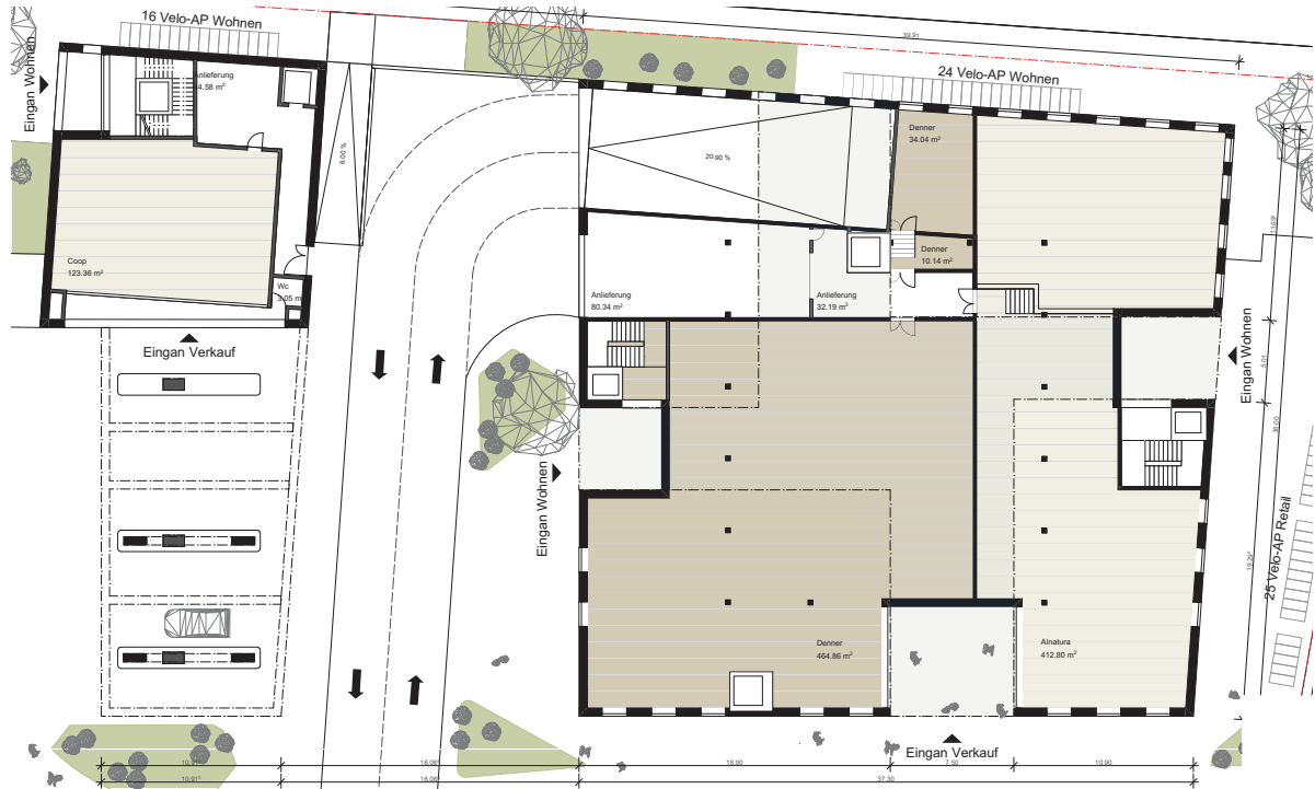
Erdgeschoss 1:200
