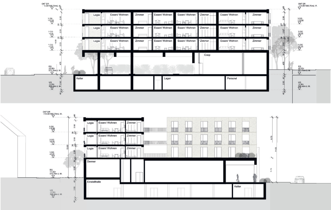
Schnitt B-B und Schnitt C-C Burckhardt + Partner AG | Köniz „Plaza“ | Projektstand 19.11.2020
